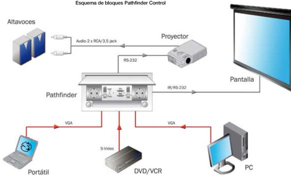
Esquema de bloques Pathfinder Control
