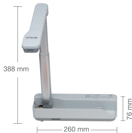
Dimensiones abierto
